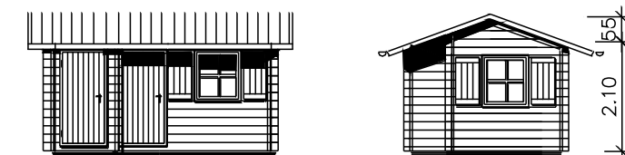
Ansichten First um 90° gedreht
