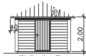
Einflügelige Tür
