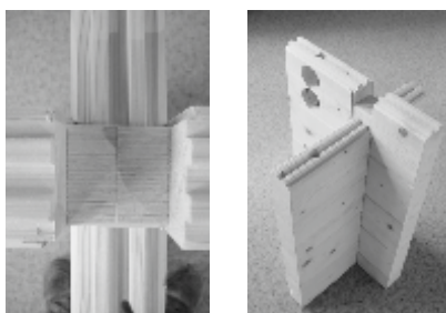
Klassische Eckverbindung
